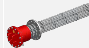
集束式法兰电加热器 Circulation Heaters
