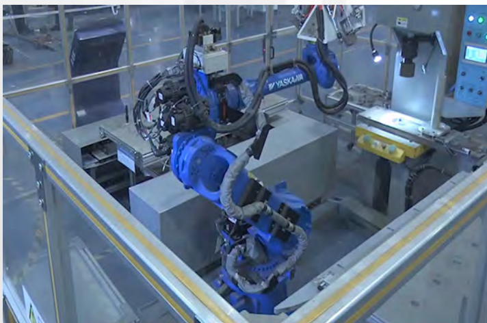
5. 自动组装 Automatic Assembly
